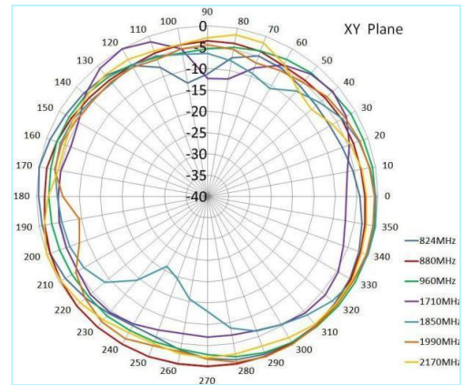
GSM部分方向图
