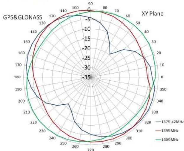
GPS Antenna
