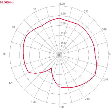
Horizontal 6000.000MHz
