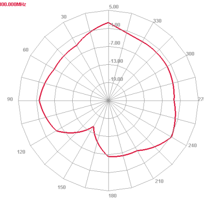
Horizontal 5800.000MHz
