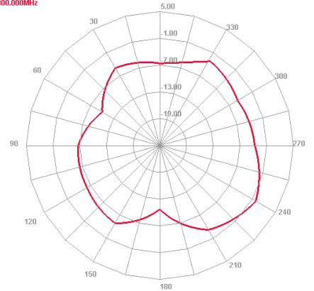
4800.000MHz
