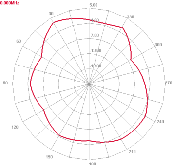
E2 Face 5800.000MHz
