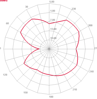
Horizontal 2400.000MHz
