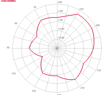
Horizontal 2600.000MHz
