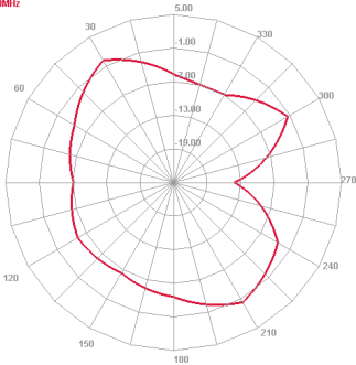
E2 Face 2400.000MHz
