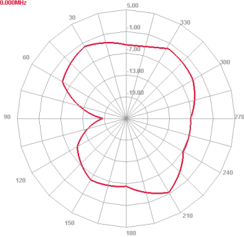
E2 Face 2400.000MHz
