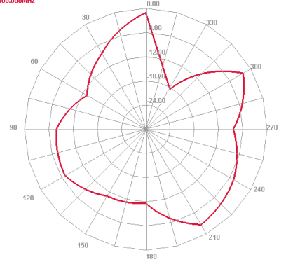
E2 Face 4800.000MHz
