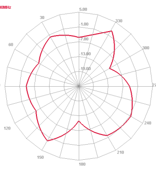
Horizontal 2600.000MHz
