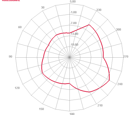
E2 Face 4800.000MHz
