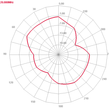
Horizontal 7120.000MHz
