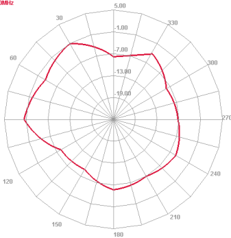
Horizontal 3500.000MHz
