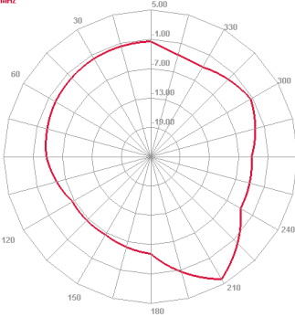
E2 Face 2600.000MHz
