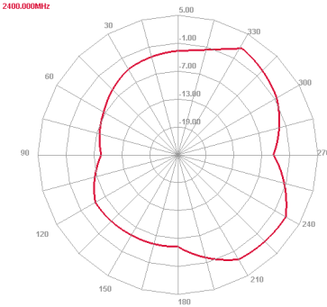
Horizontal 2400.000MHz
