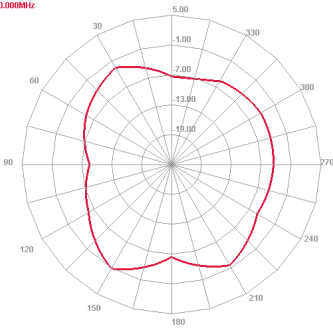
E2 Face 2400.000MHz
