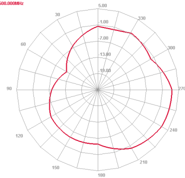
Horizontal 3500.000MHz
