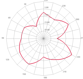
Horizontal 2400.000MHz
