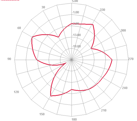
4800.000MHz
