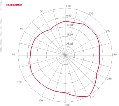
Horizontal 4800.000MHz
