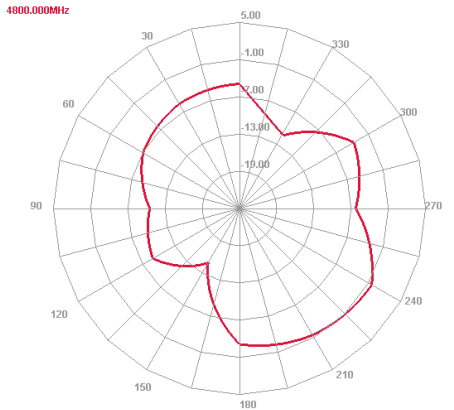
Horizontal 4800.000MHz
